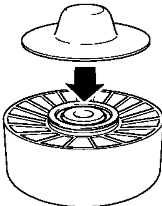
Nosný valček s plastickým krytom pre drážkovaný klinový remeň.
